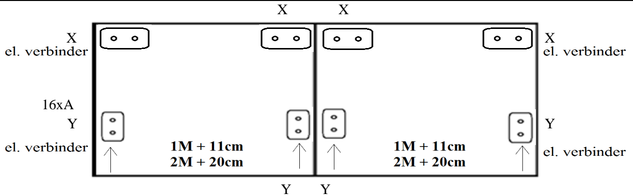
Element zonder arm: 2 zits Relax/ 2,5 zits Relax/ 3(2x90) zits Relax
